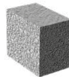
L x B x H in cm: 30,0 x 17,5 x 24,8 Ergänzungsstein
