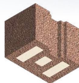
L x B x H in cm: 24,7 x 36,5 x 24,9 12 DF Endstein Nut
